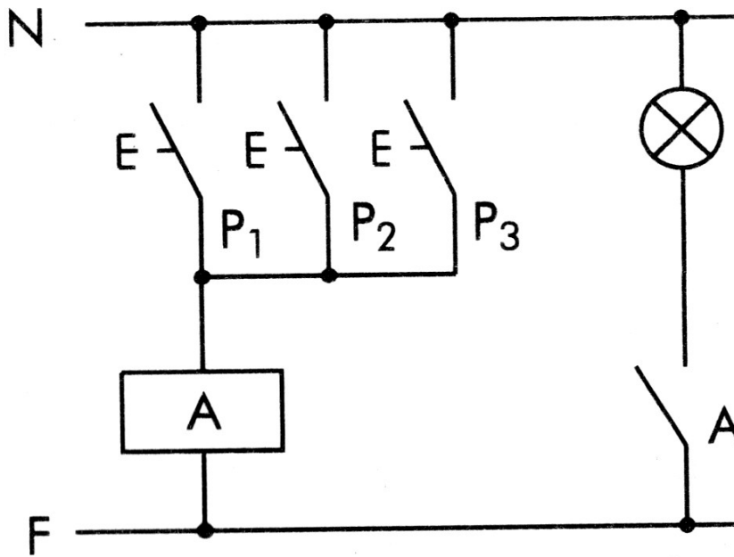
Impianto luce con relè interruttore
