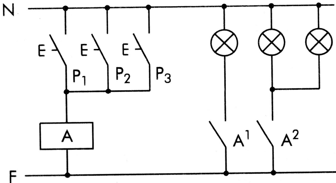
Impianto luce con relè commutatore
