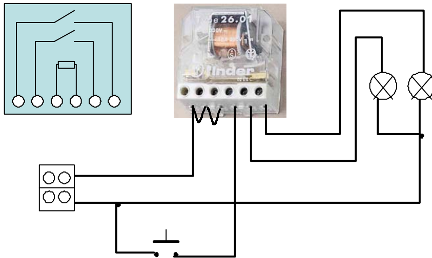
Schema di montaggio Impianto luce con relè commutatore
