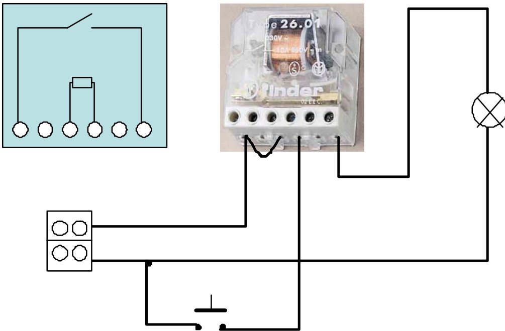
Schema di montaggio Impianto luce con relè interruttore
